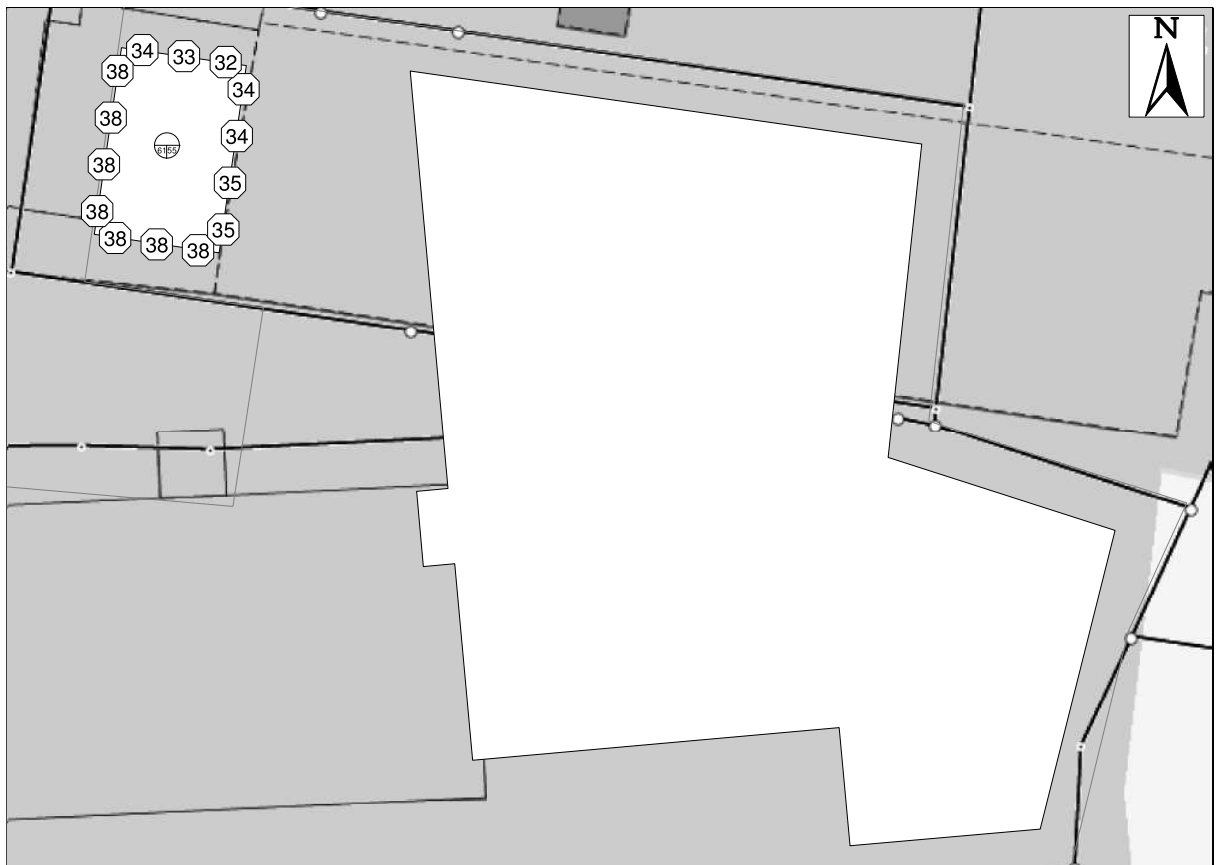
Abbildung 4 Gebäudelärmkarte: Erforderliche Bau-Schalldämm-Maße R'_{w,ges}
